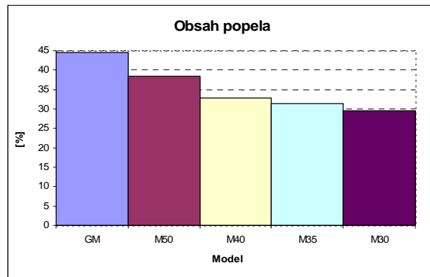
Graf 2: Průměrný obsah popela A d jednotlivých modelů.
